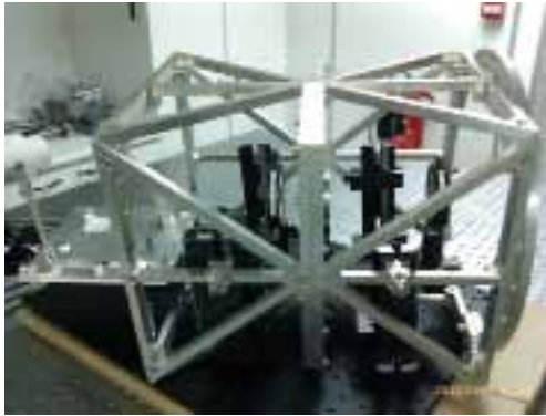
MERLIN en el Laboratorio de Óptica. Se pueden ver el tip-tilt, el espectrógrafo, la cámara, la óptica y la interfaz mecánica.
